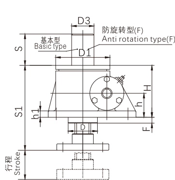
装配型式B Assembly type B
