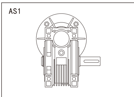
单向输出轴位置图 Position Of Single Output Shaft
